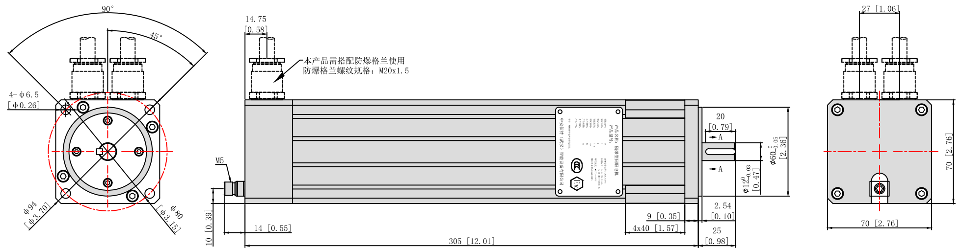
动力线端子
